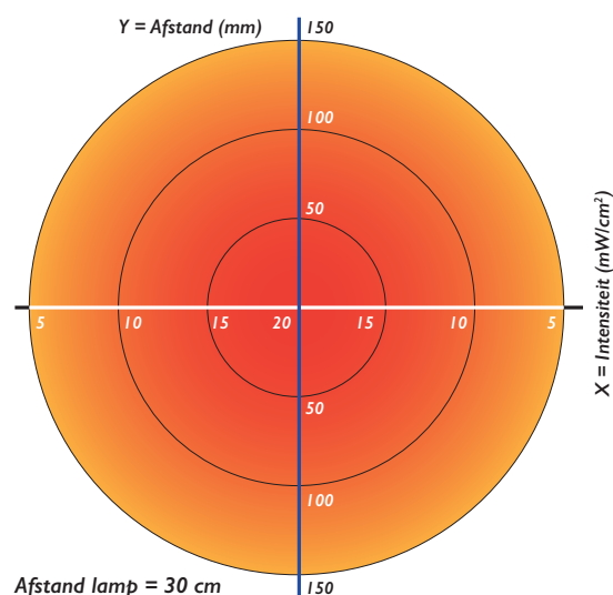
Intensiteitsgrafiek UV-A Licht (365 nm)
